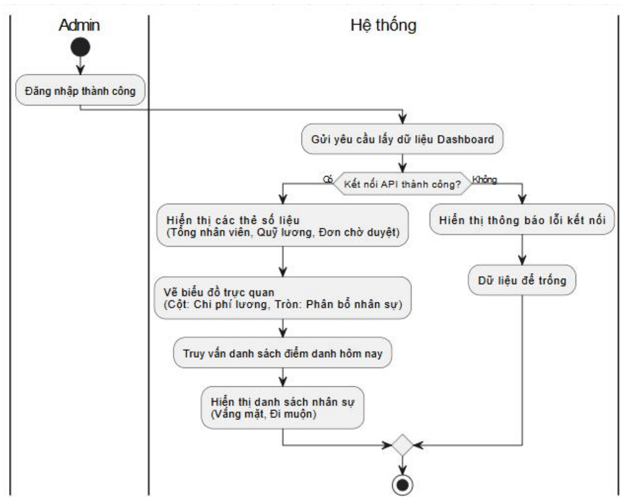
Hình 4 Biểu đồ hoạt động của dashboard admin
