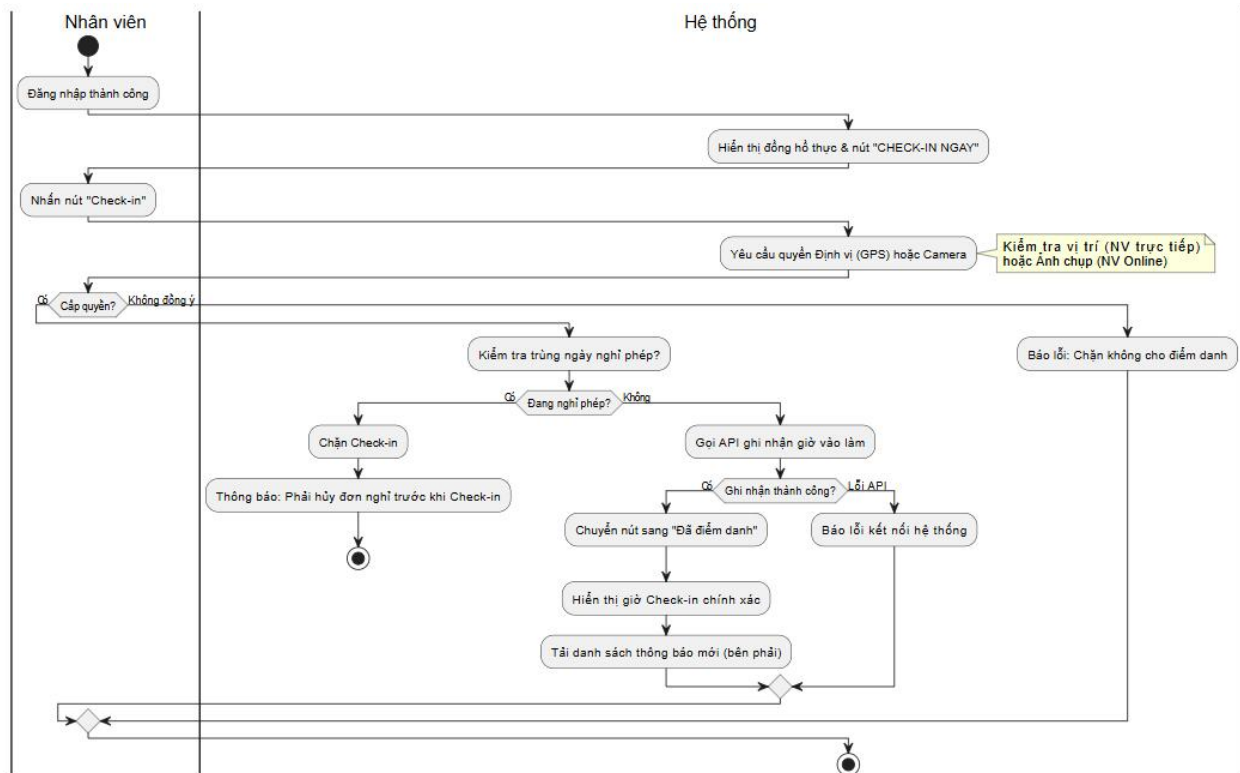
Hình 5 Biểu đồ hoạt động của dashboard nhân viên
