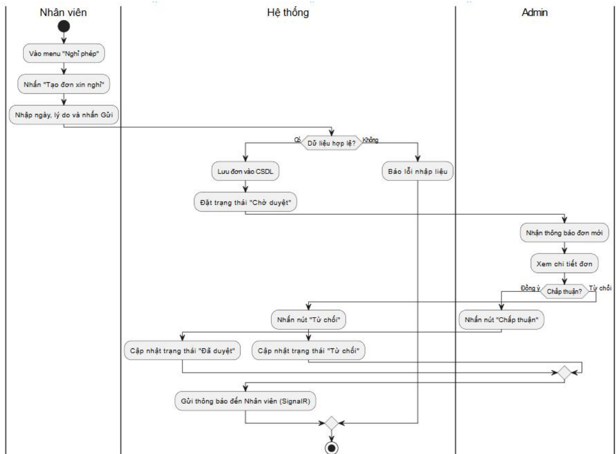
Hình 9 Biểu đồ hoạt động của quản lý nghỉ phép
