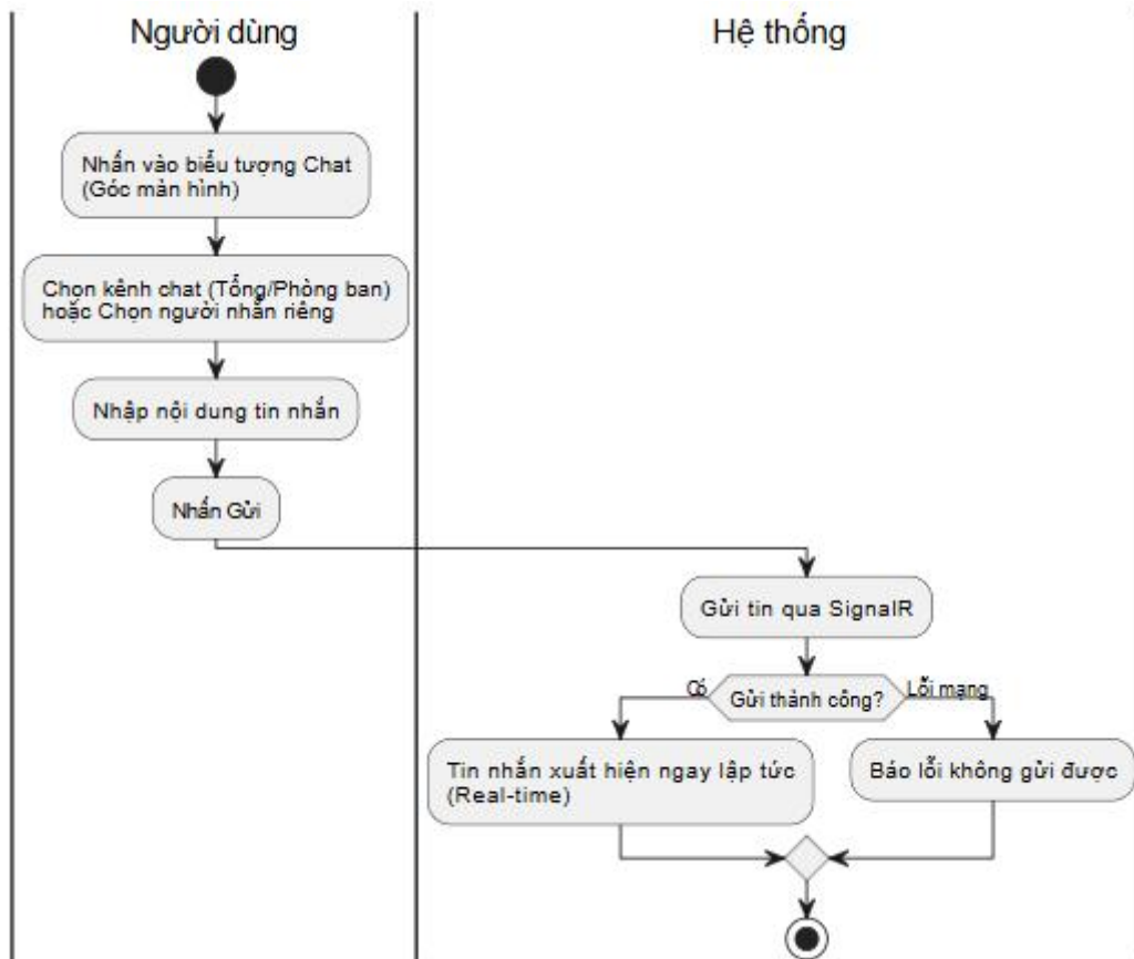
Hình 13 Biểu đồ hoạt động của tính năng kênh chat
