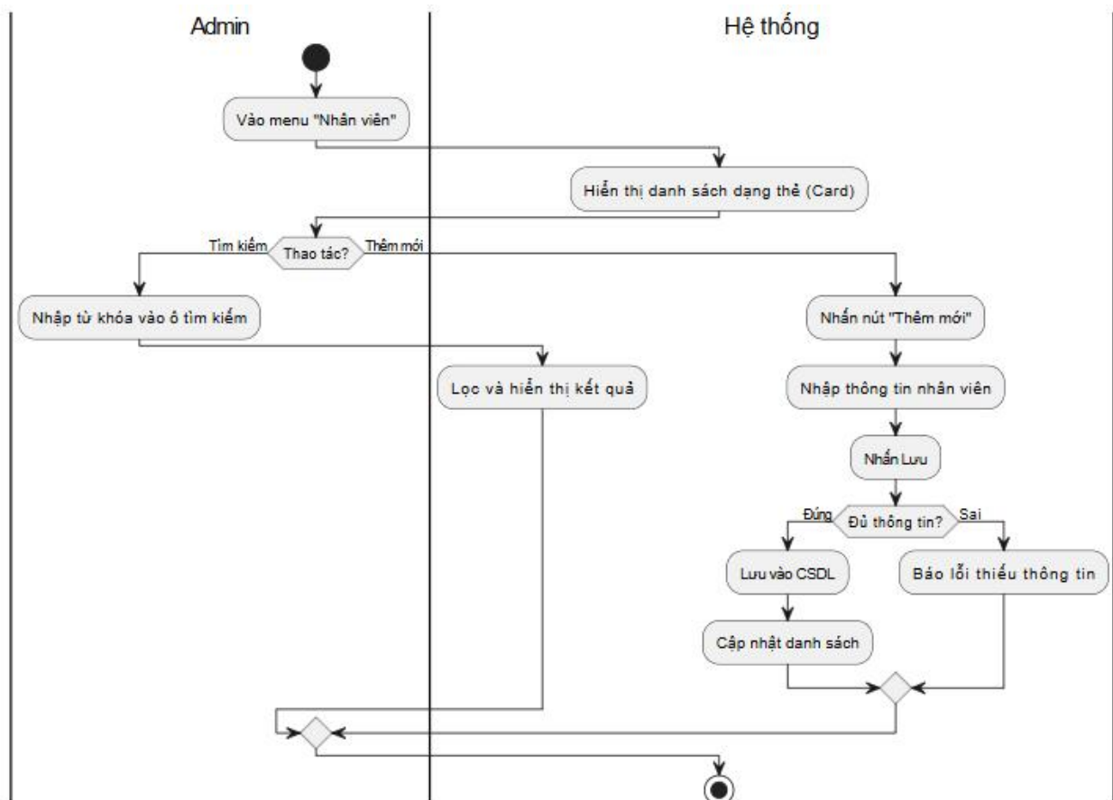
Hình 6 Biểu đồ hoạt động của quản lý nhân viên
