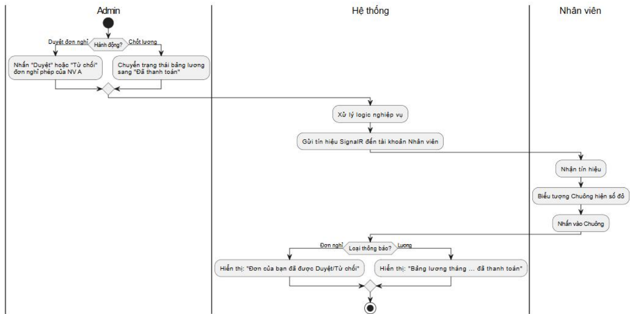
Hình 15 Biểu đồ hoạt động của tính năng chuông thông báo
