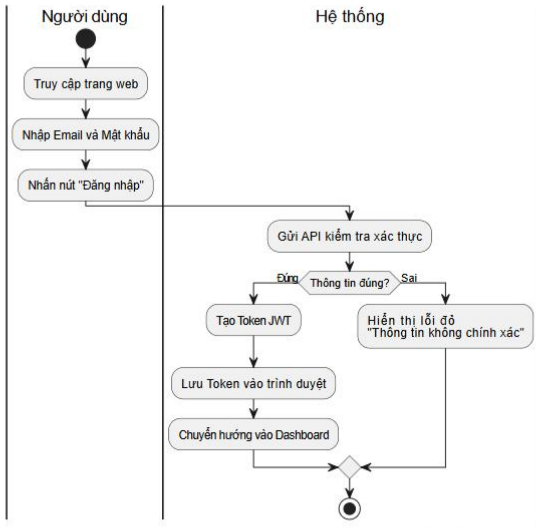
Hình 2 Biểu đồ hoạt động của đăng nhập
