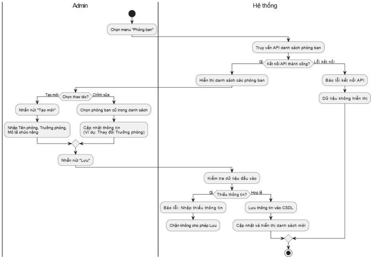
Hình 7 Biểu đồ hoạt động quản lý phòng ban
