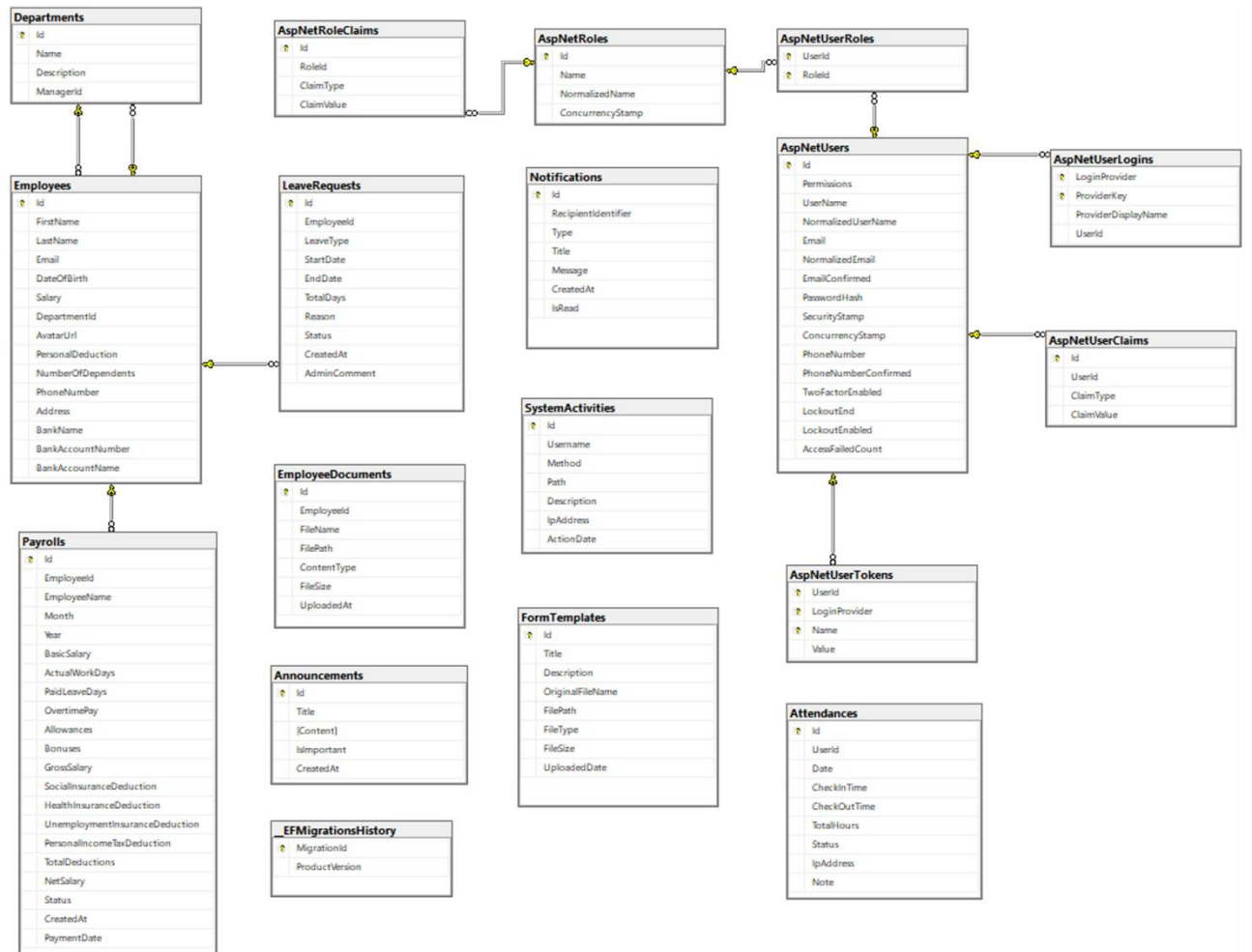
Hình 17 Sơ đồ database
