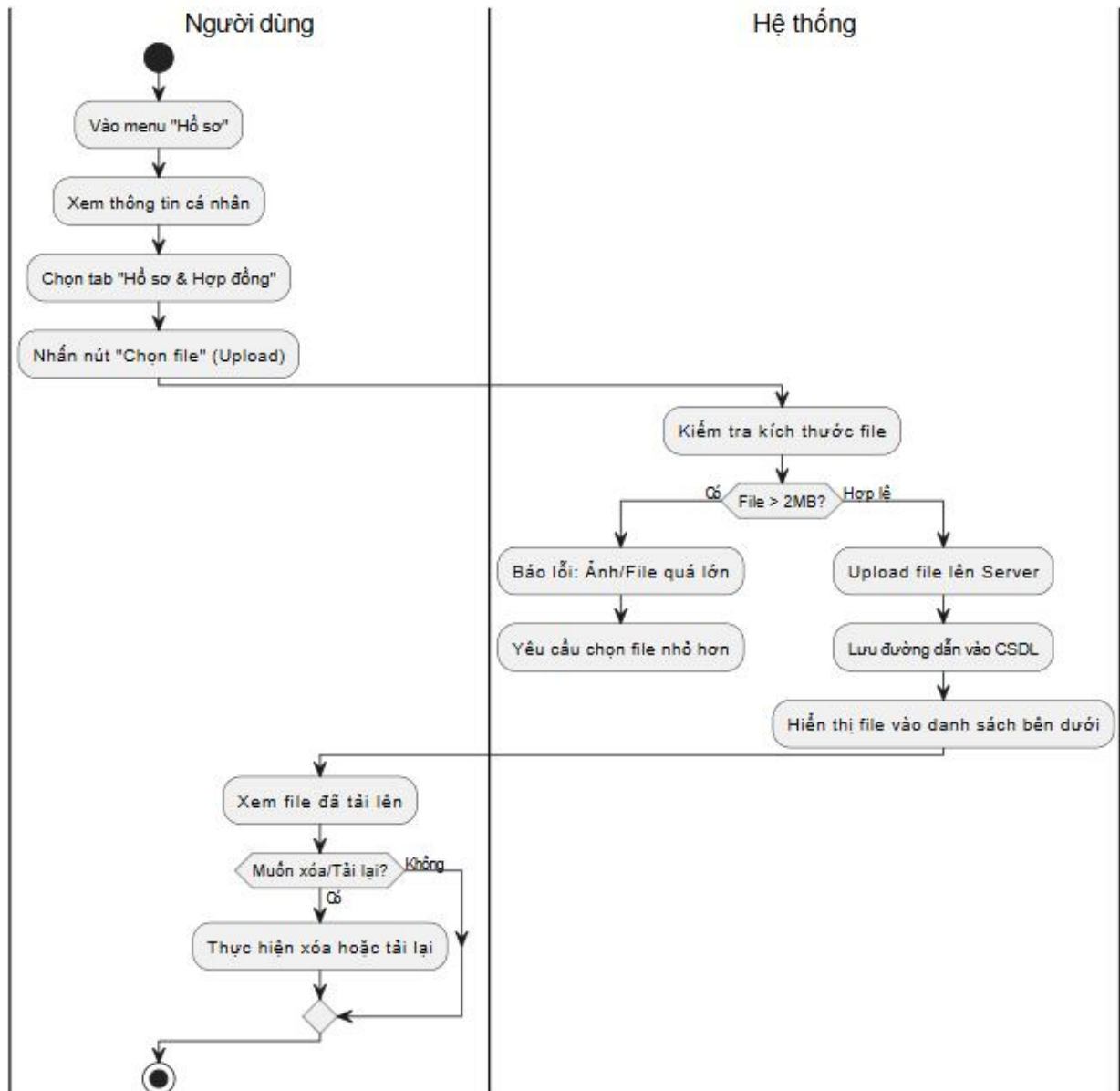
Hình 11 Biểu đồ hoạt động của quản lý hồ sơ cá nhân
