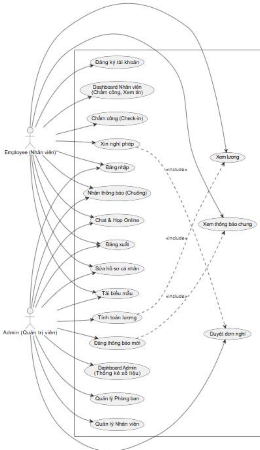
Hình 1 Biểu đồ usecase tổng quát
