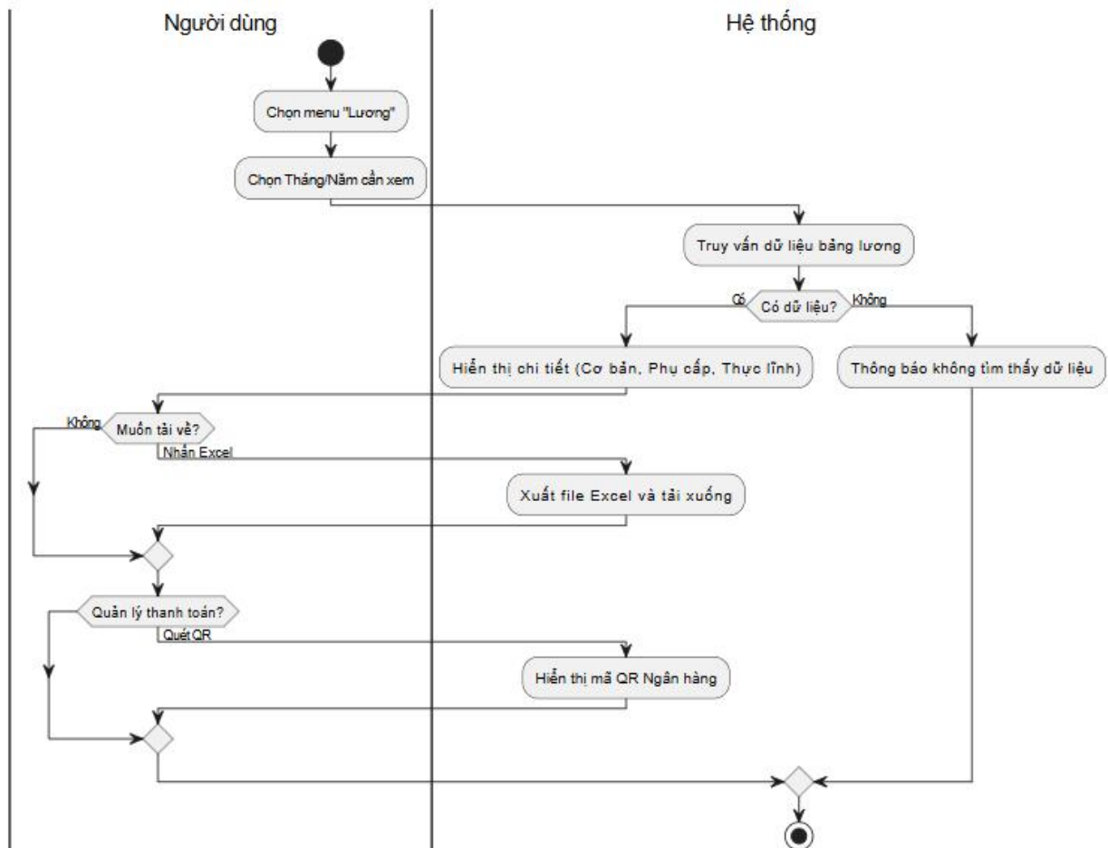
Hình 8 Biểu đồ hoạt động của quản lý lương và thưởng
