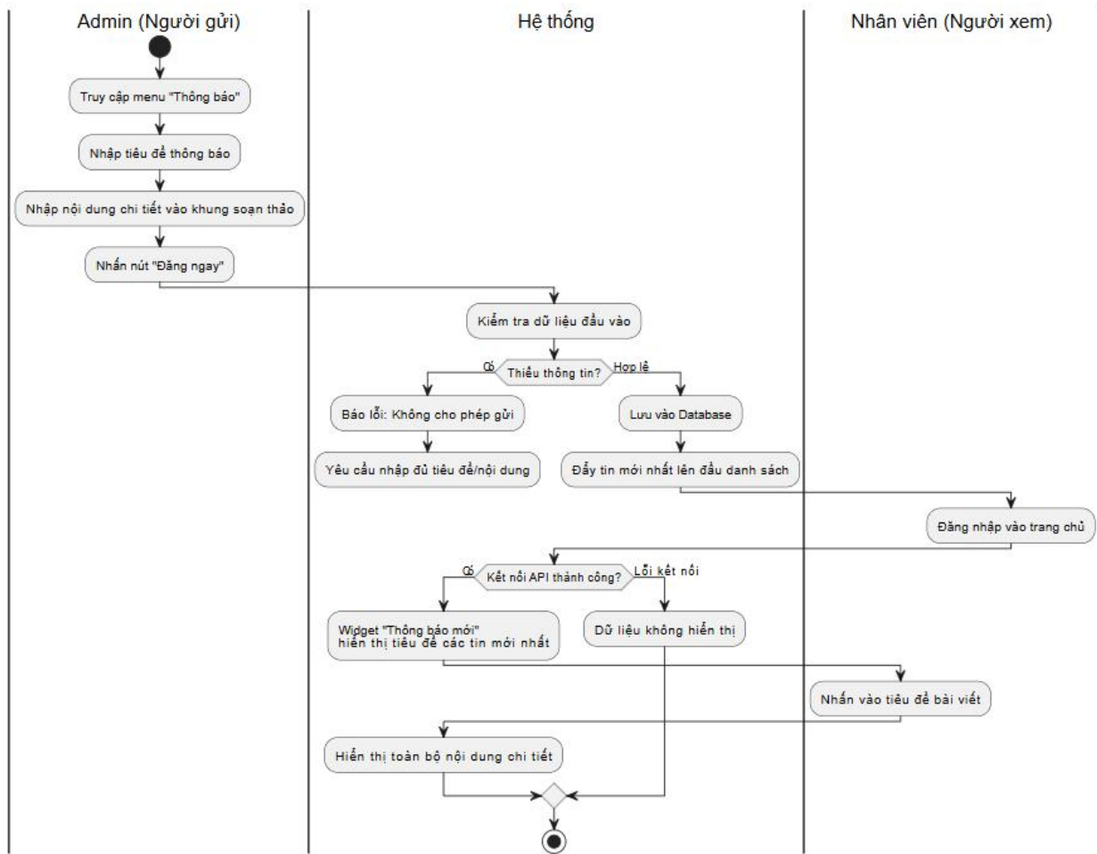
Hình 10 Biểu đồ hoạt động của quản lý thông báo chung
