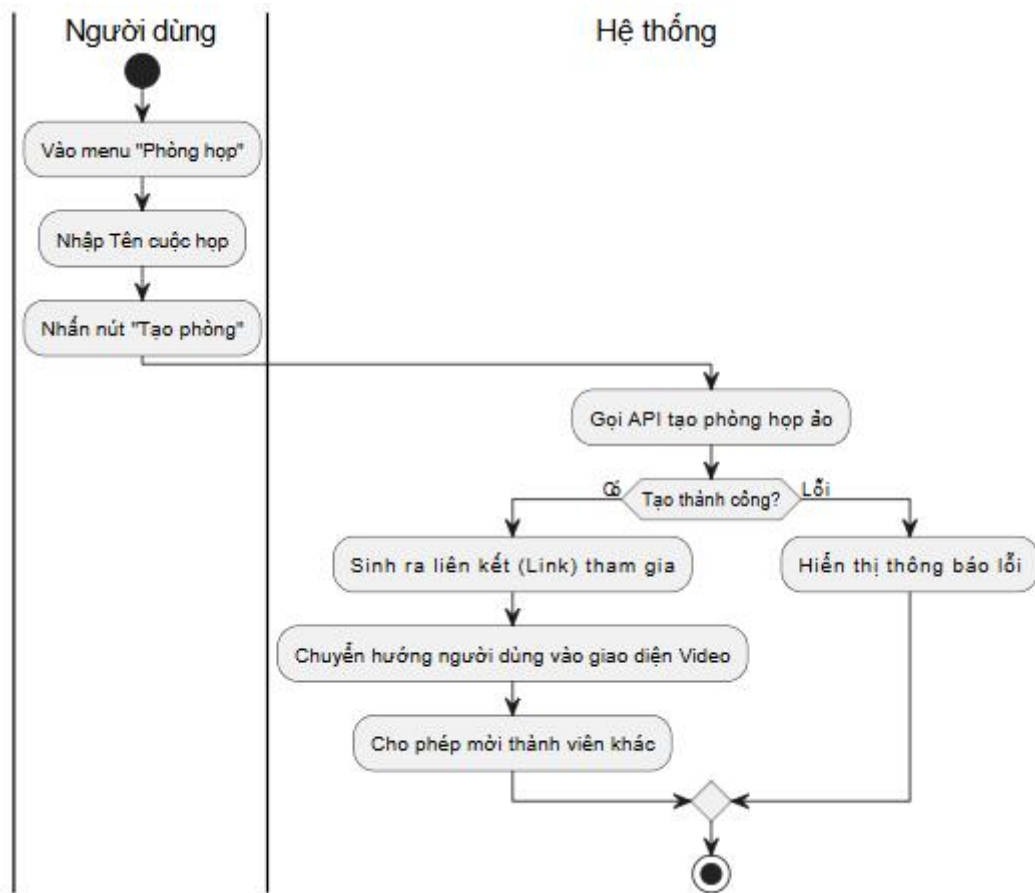
Hình 14 Biểu đồ hoạt động của tính năng phòng họp
