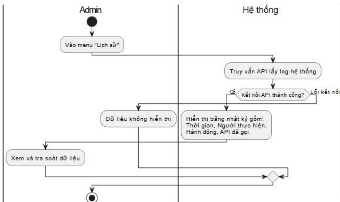
Hình 12 Biểu đồ hoạt động của quản lý nhật ký hoạt động
