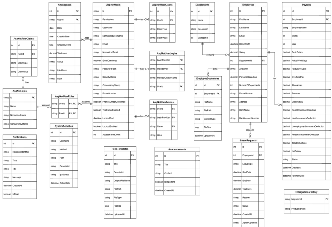
Hình 16 Sơ đồ ERD
